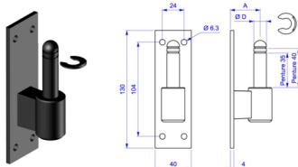
Gond sur platine court
